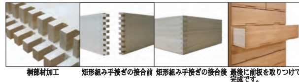
78-5段チェスト W784×D441×H1065 ¥133,000 (税込¥146,300)
